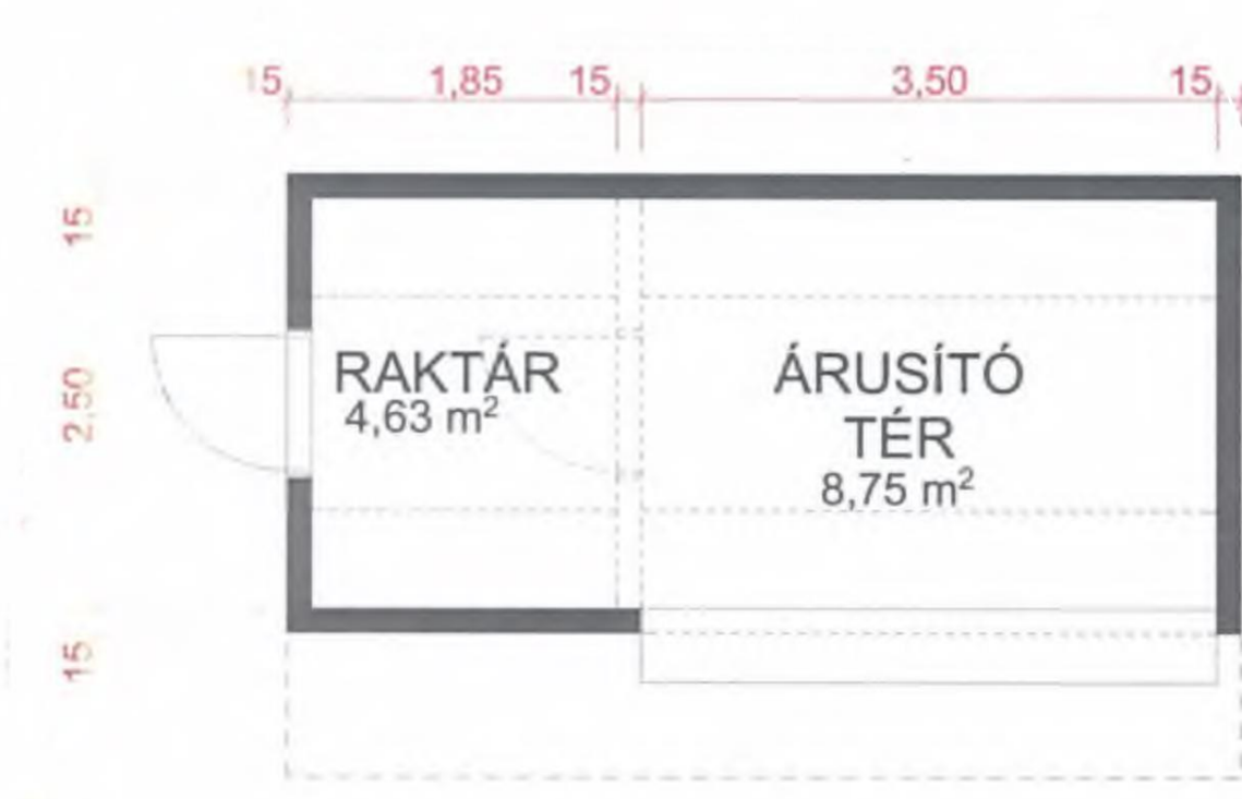
pavilon alaprajz
